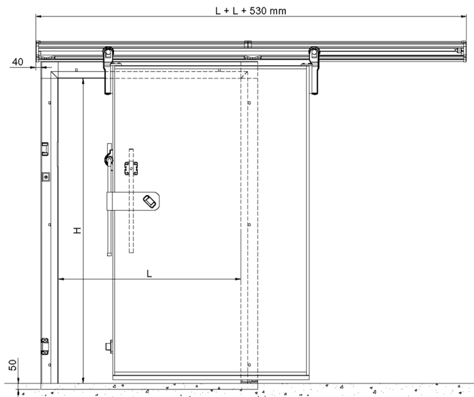
L = Largeur de passage libre H = Hauteur de passage libre
